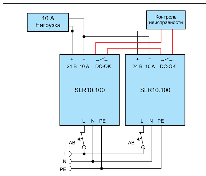
Рис. 11. Схема резервирования, построенная на ИП серии SLR10 со встроенной схемой развязки
