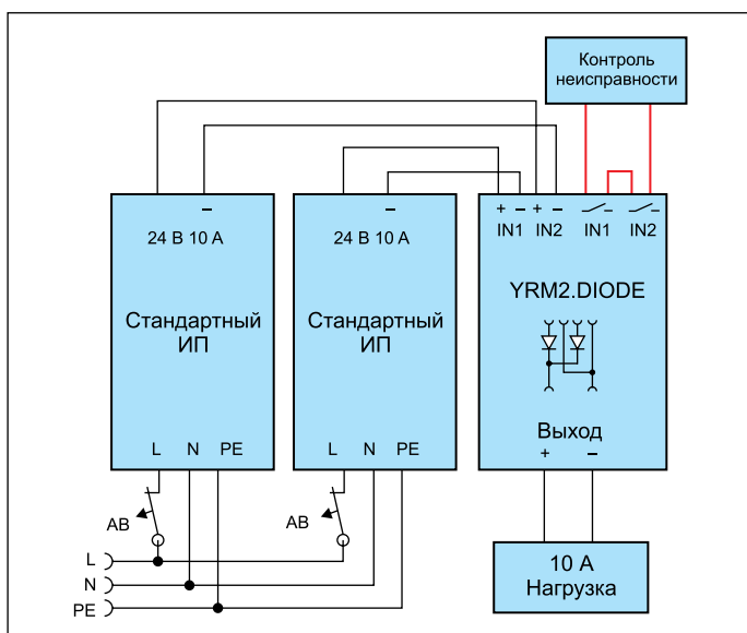
Рис. 10. Схема резервирования стандартного ИП с помощью диодного модуля YRM2.DIOD
