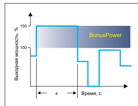
Рис. 4. График гарантированного 150%-го запаса по мощности ИП серии Q
