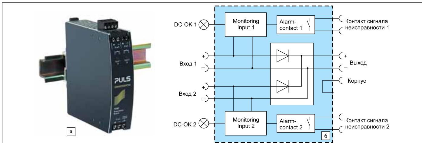
Рис. 9. а) Развязывающий диодный модуль YRM2.DIOD; б) его функциональная схема
