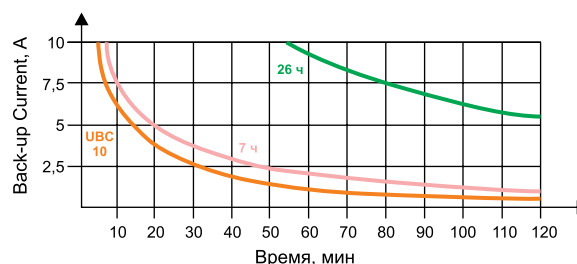
Рис. 8. Типовые бэкап-характеристики: с внешним аккумулятором UBC10 со встроенным аккумулятором 5 А·ч (оранжевая кривая), с внешним аккумулятором 7 А·ч (розовая кривая), с внешним аккумулятором 26 А·ч (зеленая кривая)
