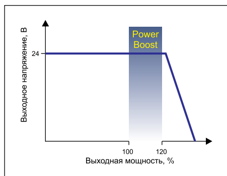
Рис. 1. График выходной мощности для ИП серии C
