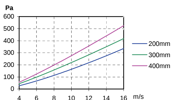
Druckverlust / pressure drop
