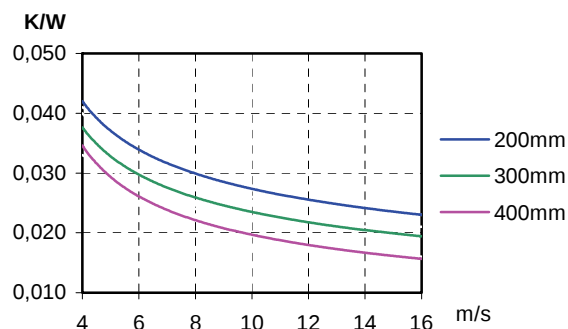
Thermischer Widerstand / thermal resistance
